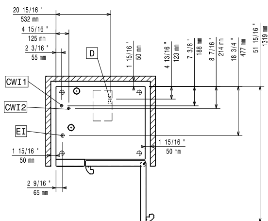
Boven aanzicht
